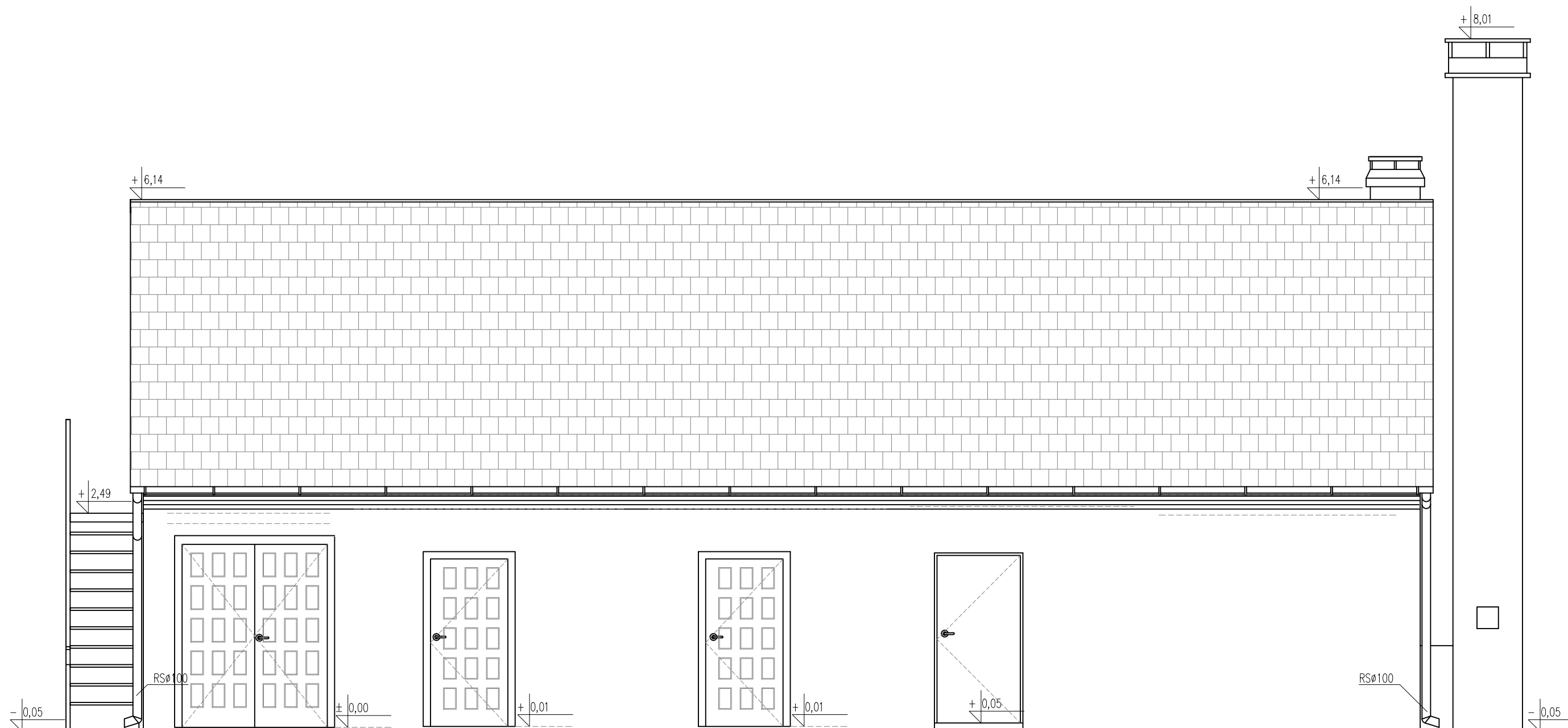
ELEWACJA WSCHODNIA (FRONTOWA) SKALA 1:50
