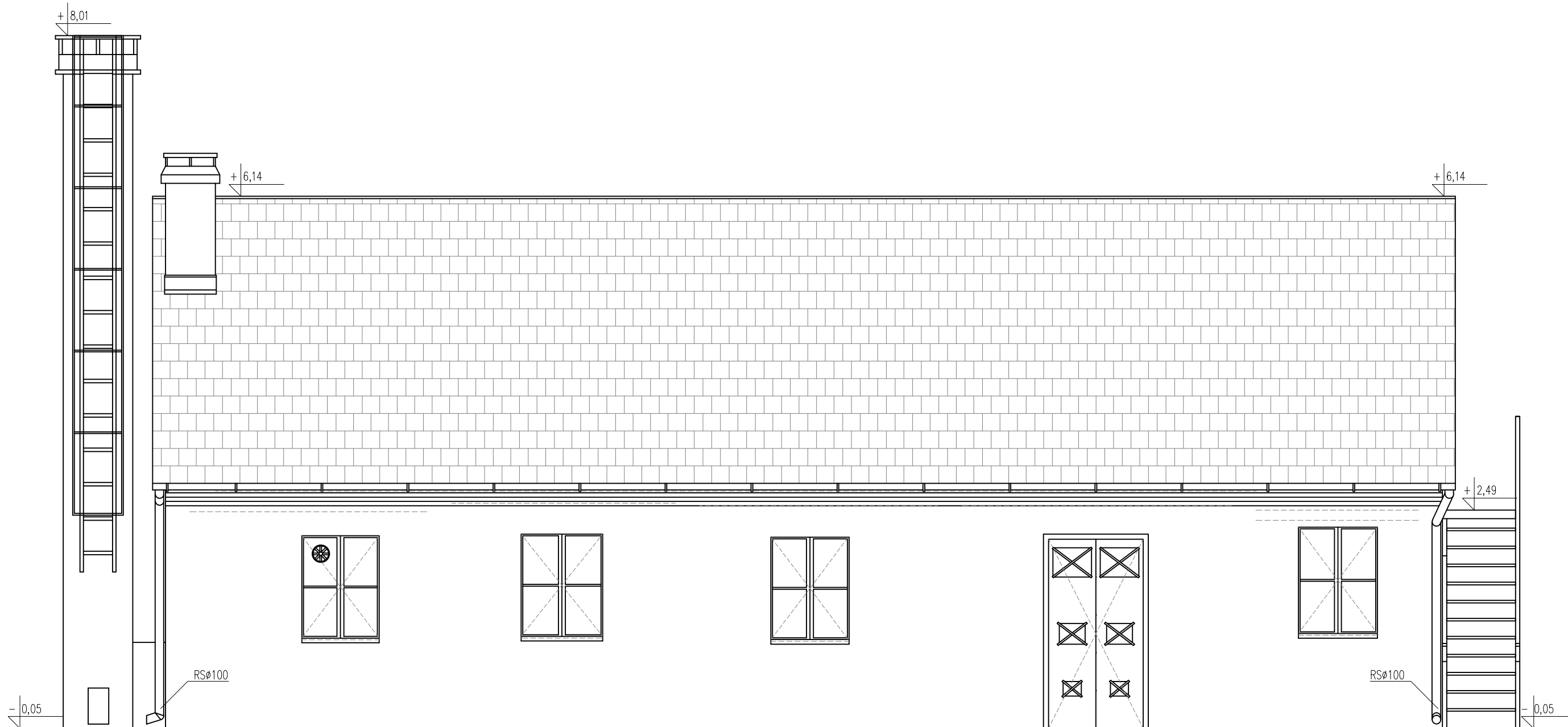
ELEWACJA ZACHODNIA (TYLNA) SKALA 1:50
