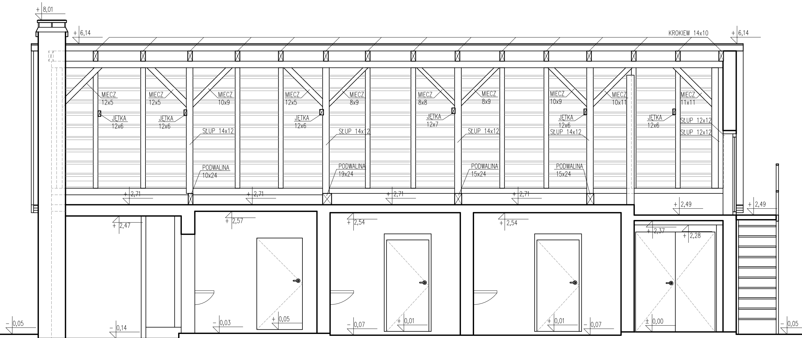
PRZEKRÓJ A-A SKALA 1:50
